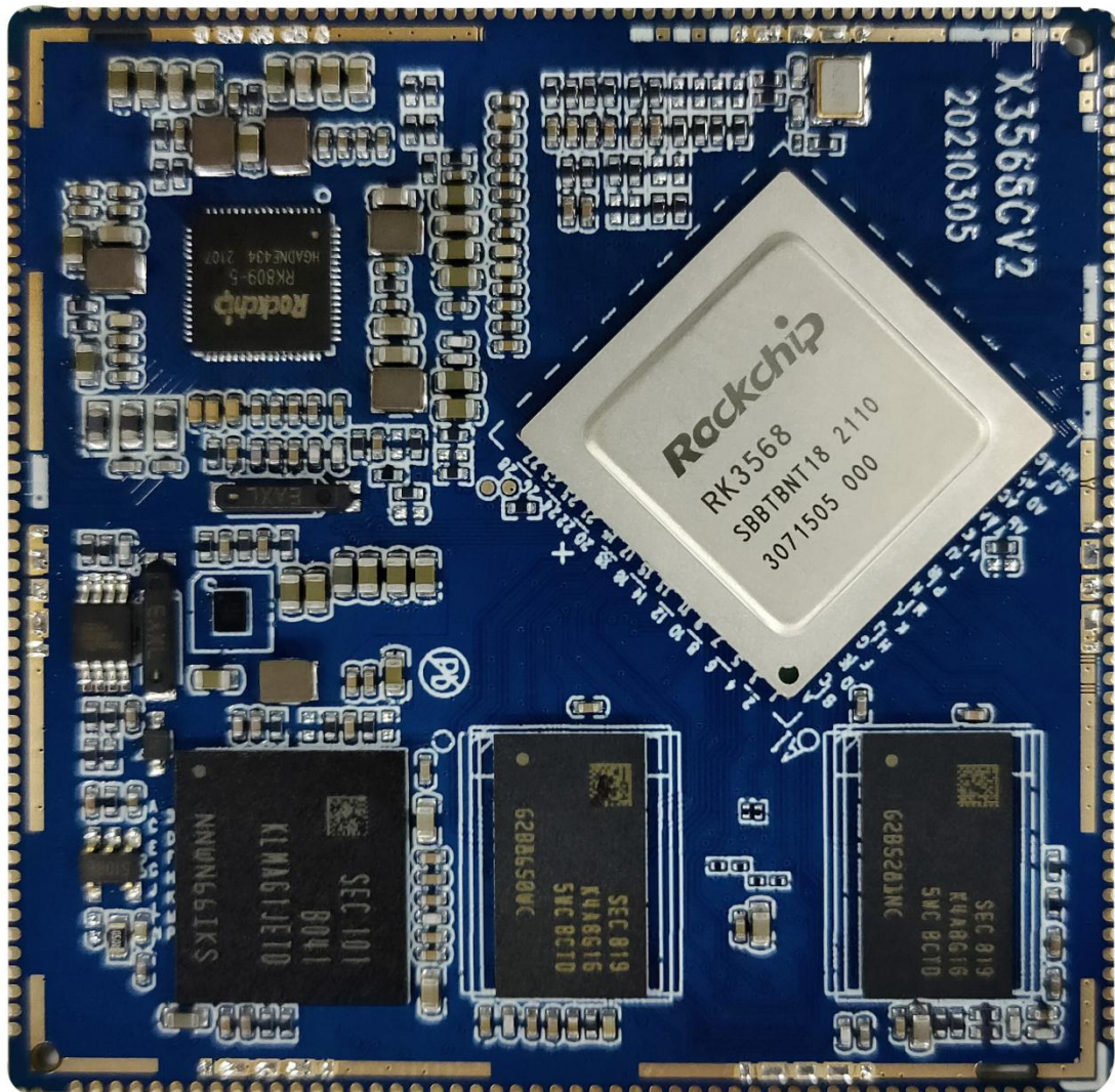
核心板正面图
